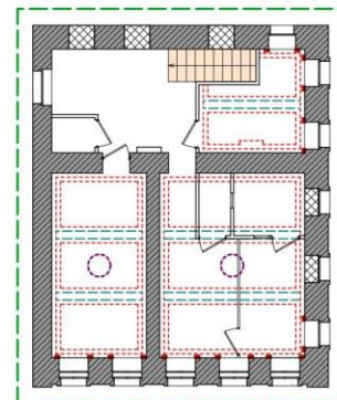
План-схема 2 этажа
